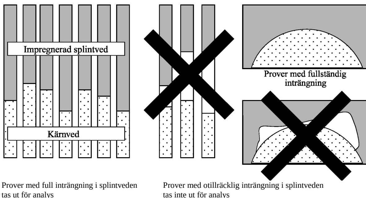
Figur 10.3 Prover som uttas för analys av upptagningen.
