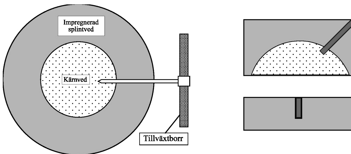
Figur 10.1 Exempel på uttag av borrprover från rundvirke och sågat virke.
