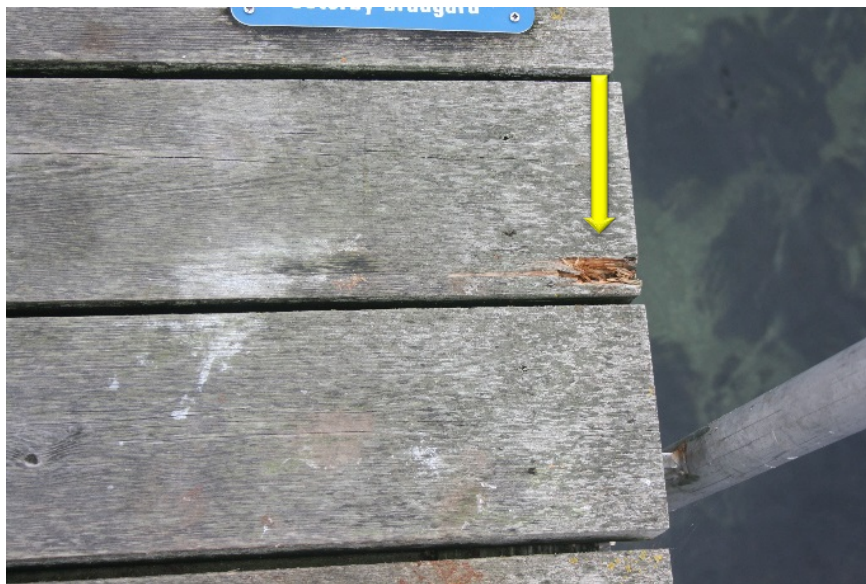
Figur 11. Brunröteangrepp i planka av gotländsk furukärnved behandlad med Sioo. Angreppet har skett i splintved. Förekomst av splintved är inte helt ovanligt i det som marknadsförs som kärnved.
