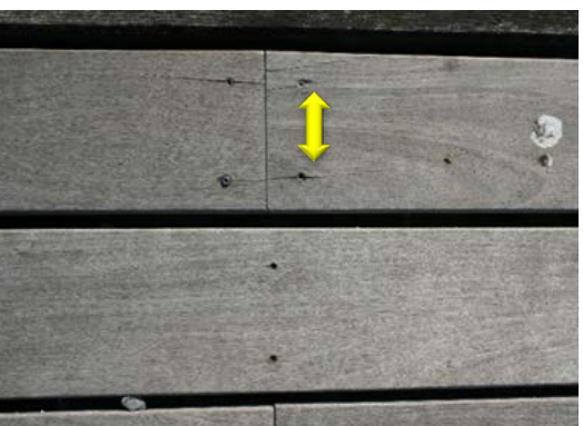
Ipé med sprickor kring skruvskallar Foto från inspektionen i oktober 2018
