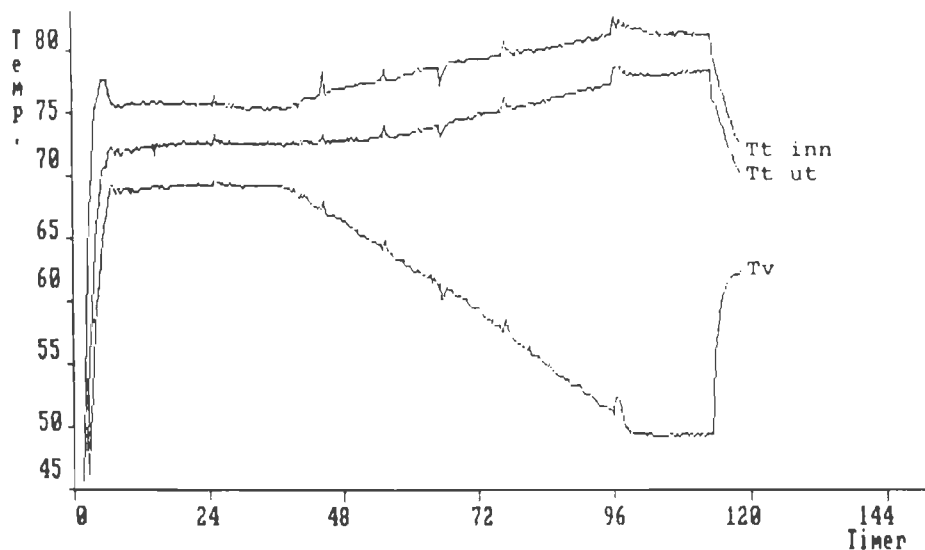
Figur 5. Registrert klima ved Forsøk nr 2 (skarpt)
