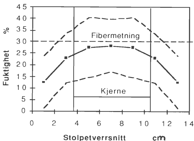
Figur 9. Midlere fuktighetsgradient etter tørking med angivelse av 90% konfidensintervall ved Forsøk 2 (skarp)
