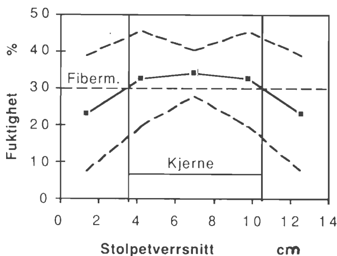
Figur 8. Midlere fuktighetsgradient etter tørking med angivelse av 90% konfidensintervall ved Forsøk 1 (mild)
