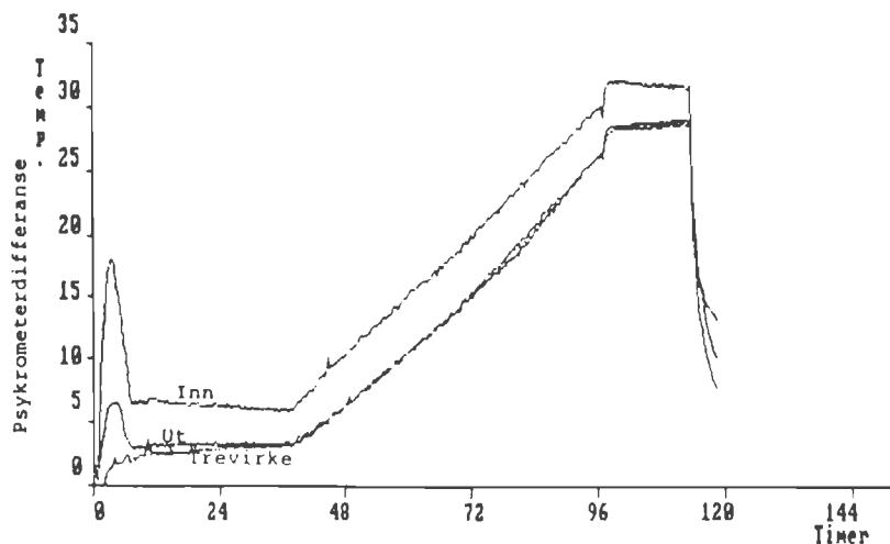
Figur 6. Psykrometerdifferanser for tørkeluft og virkesoverflate for Forsøk nr 2
