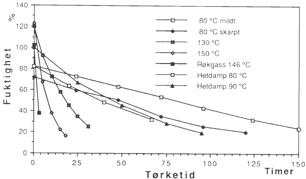
Figur 17. Registrerte tørkehastigheter avhengig av tørkeklima og tørkemetode for stolper av 15-16 cm. midlere diameter (stipulerte forløp mellom start- og slutfuktighet for 130°C, 150°C og hetdamp)
