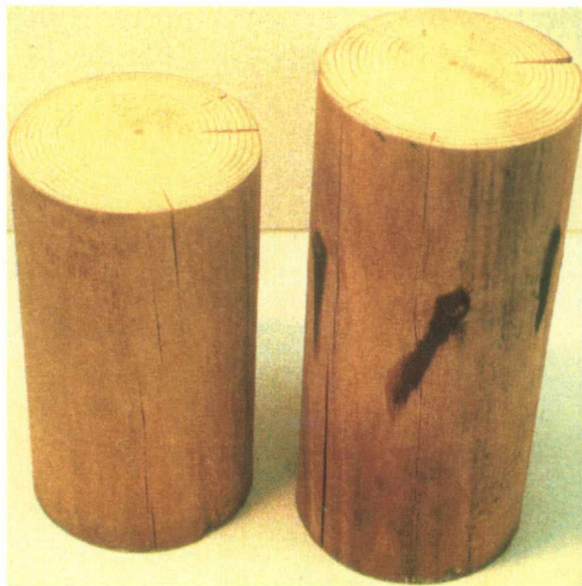
Figur 28. Sprekkbilde, kvaeflyting og fargeendring i stolper tørket ved 150°C
