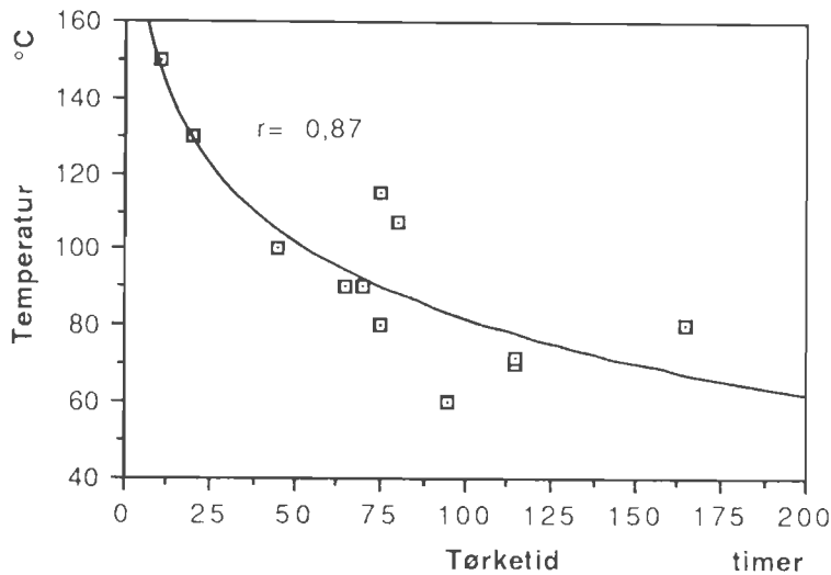
Figur 18. Sammenstilling av tørketemperaturer og tørketider (fra ca. 100% til 25% fuktighet) ved egne (eks. varmdamp) og refererte stolpetørkeforsøk med en logaritmisk kurvetilpasning (diameter fra 15-20 cm)
